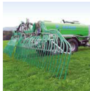
Distribuidor de manguera de arrastre Sistema modular para todo tipo de camiones cisterna
